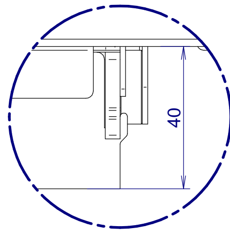
DETAIL A 1:1
