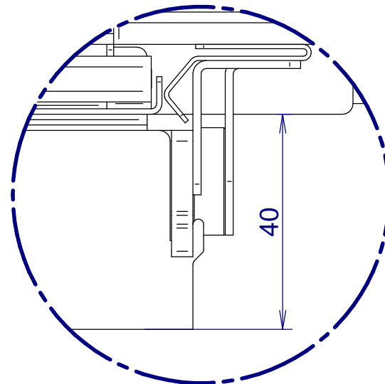
DETAIL A 1:1
